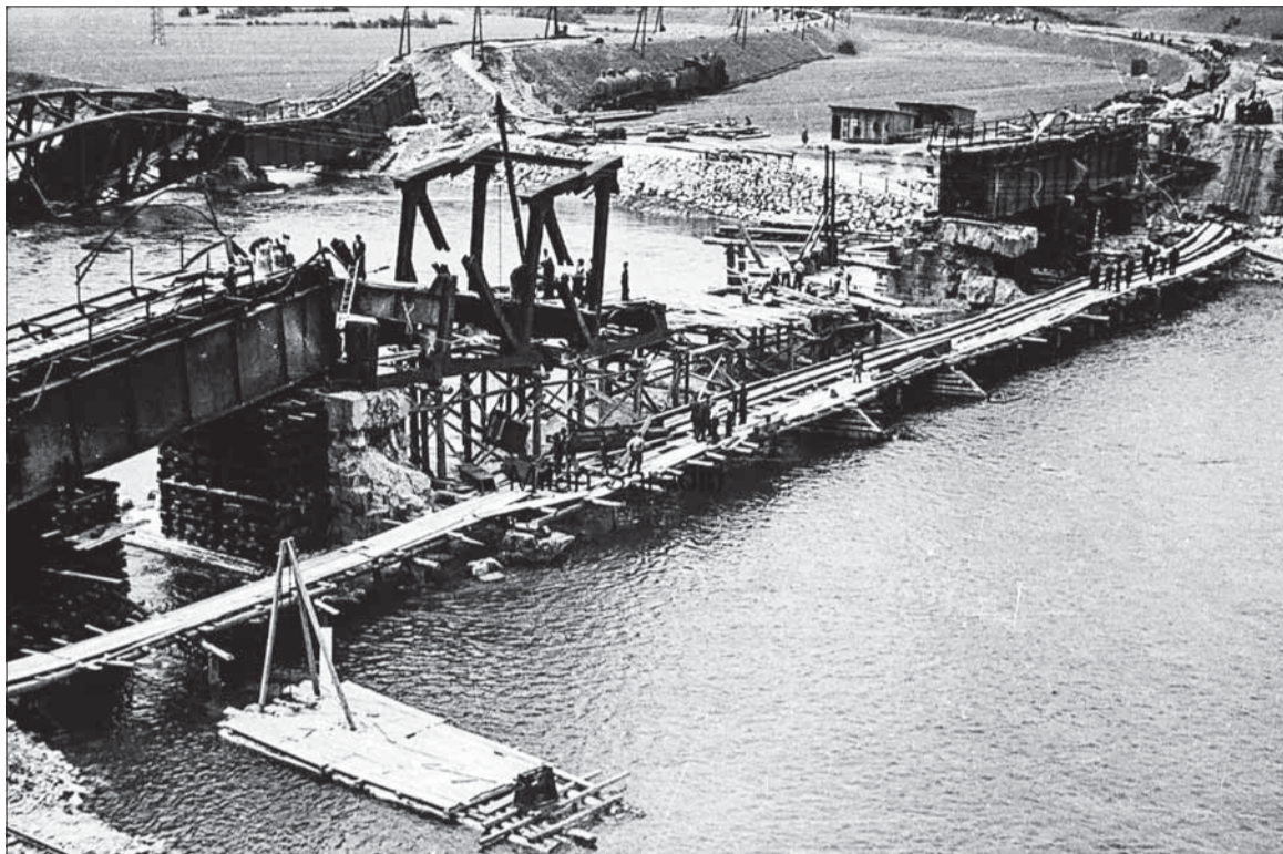
Strečno, stavba provizórneho železničného mosta.
