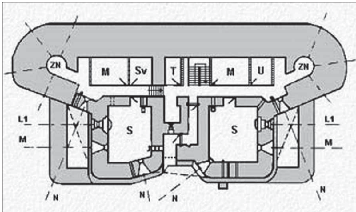
Schéma horného bojového poschodia zrubu N-S 71 – S – strelecká miestnosť, M – muničný sklad, Sv – stanovište veliteľa, T – telegrafista, U – ubikácie, ZN – zvon pre ľahký guľomet.
